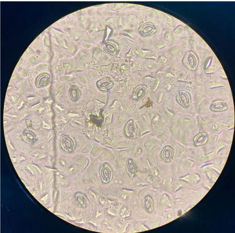
Ilustracion 18. Estomas de Avicennia germinans en 40x
