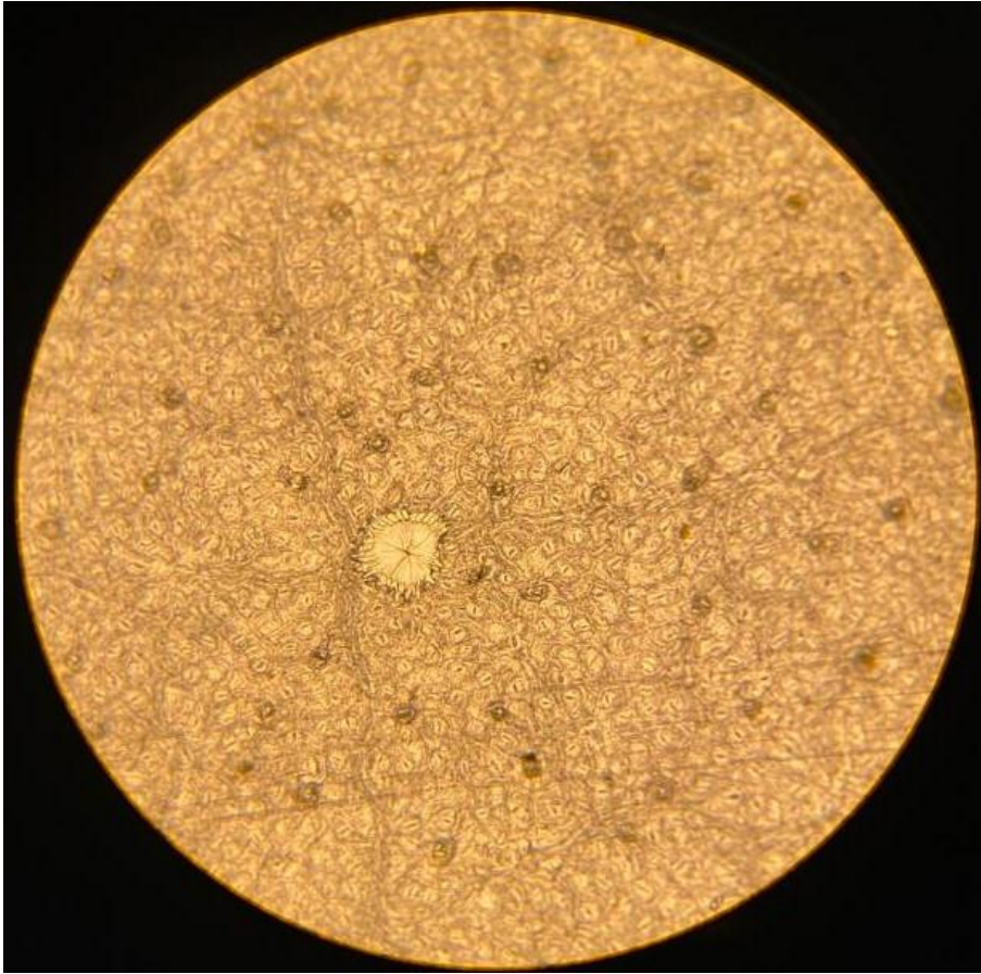
Ilustracion 8. Frutos de Thespesia populnea.
