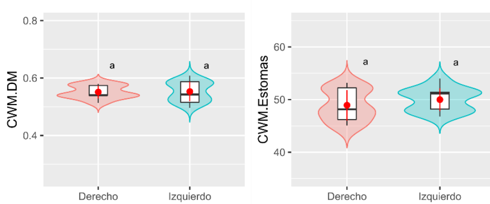
Figura 9 Media ponderada de la comunidad (CWM) para DM Y ESTOMAS.
