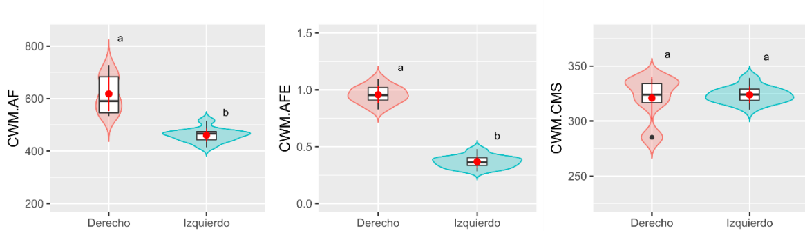
Figura 8 Media ponderada de la comunidad (CWM) para AF, AFE Y CMS.
