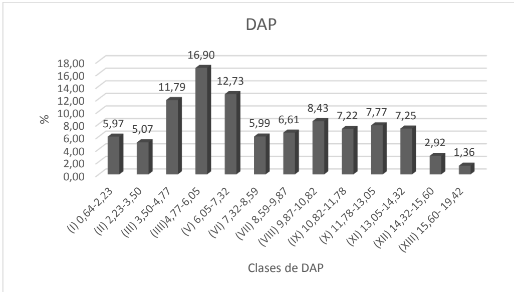
Figura 3 Grafica 3 estructura vertical lado derecho DAP
