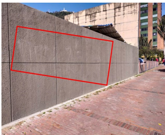
Ilustración 57 Afectación del texturizado en Graniplast aplicado en el muro de cerramiento perimetral. Fuente: Propia.
