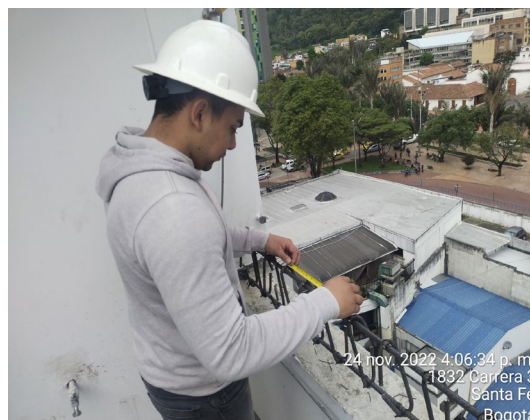
Ilustración 41 verificación de los espaciamientos del acero transversal en vigüeta. Fuente: Propia.
