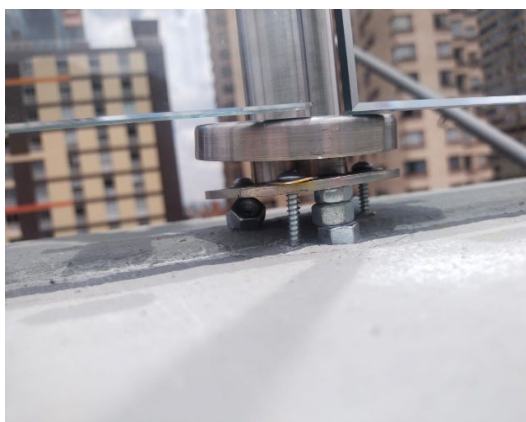
Ilustración 34 proceso constructivo de anclaje de cerramiento en vidrio incorrecto. Fuente: Propia.
