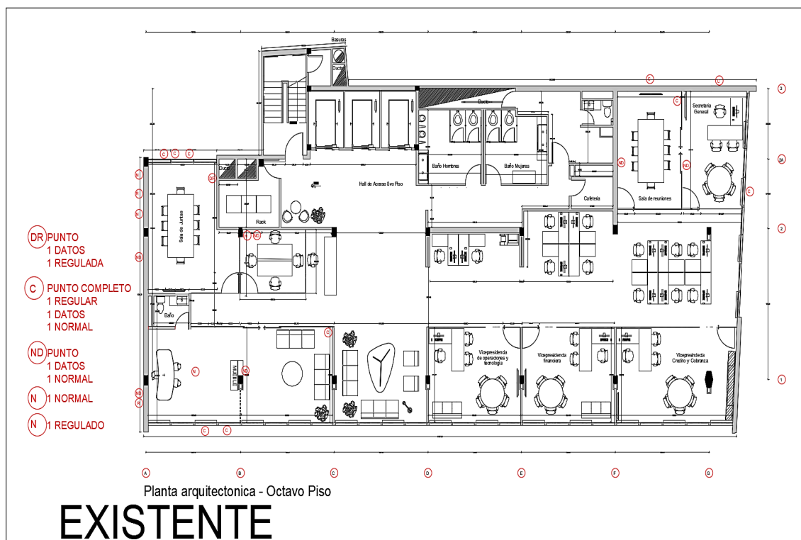
Ilustración 63 Plano con las conexiones de voz y datos existentes. Fuente: Propia
