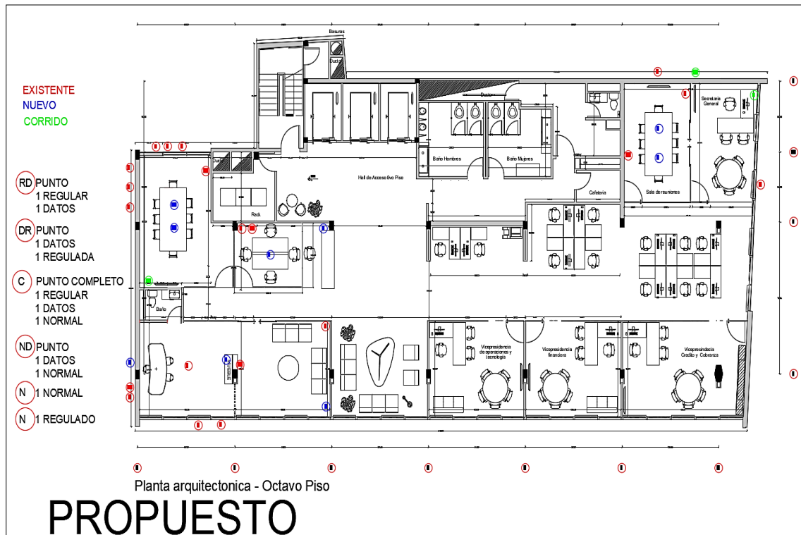
Ilustración 64 Plano con las conexiones de voz y datos necesarias para garantizar la conectividad de los espacios. Fuente: Propia.
