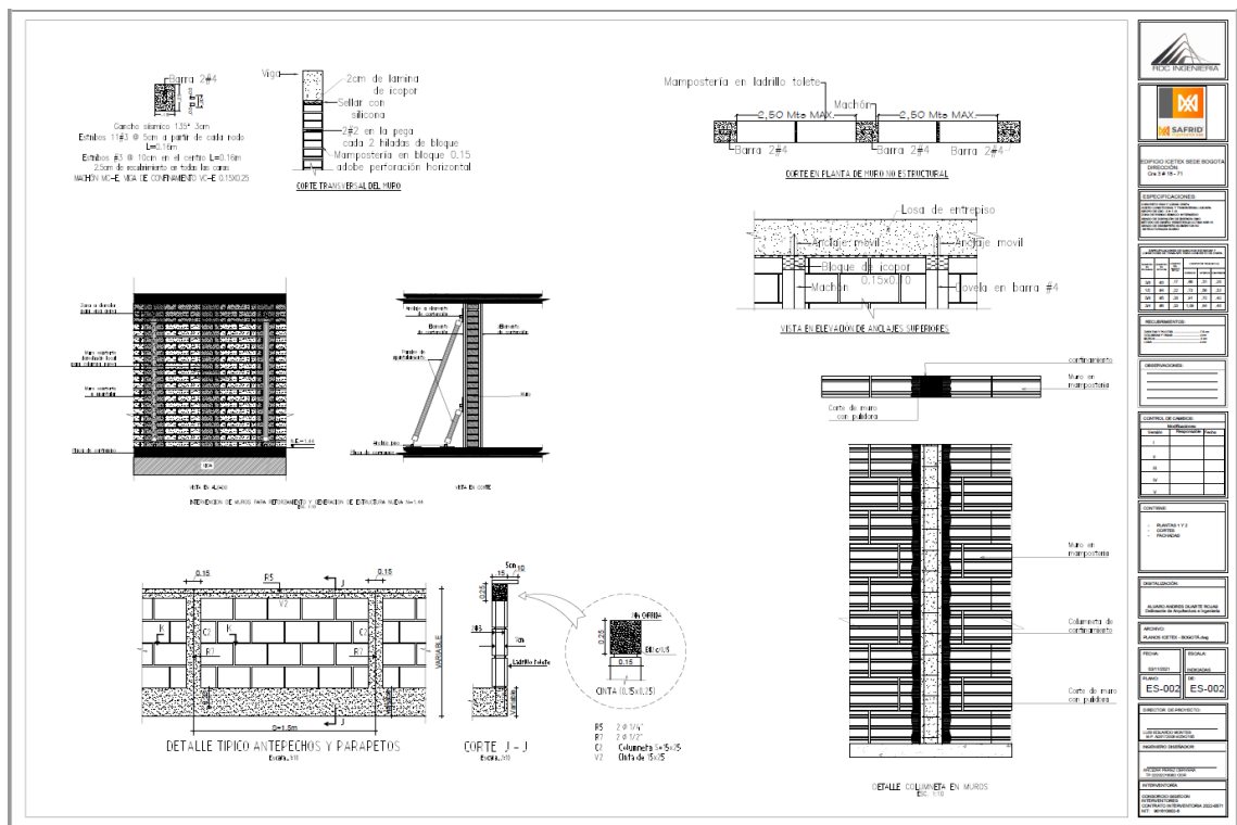
Ilustración 38 Plano Estructural Viga cinta para Cerramiento en vidrio terrazas piso 9 y piso 2. Fuente: (SAFRID, 2022)
