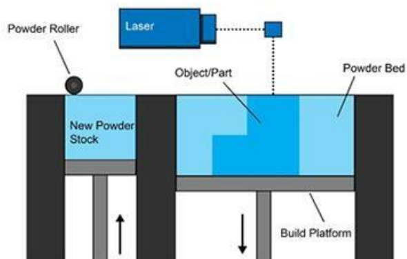
Figura 3. Proceso de fusión de lecho de polvo. Powder bed fusión. Fuente: (Loughborough, 2019)
