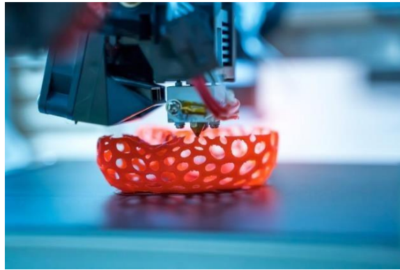
Figura 1. Funcionamiento de impresión 3D por Método de Extrusión Fundida.
