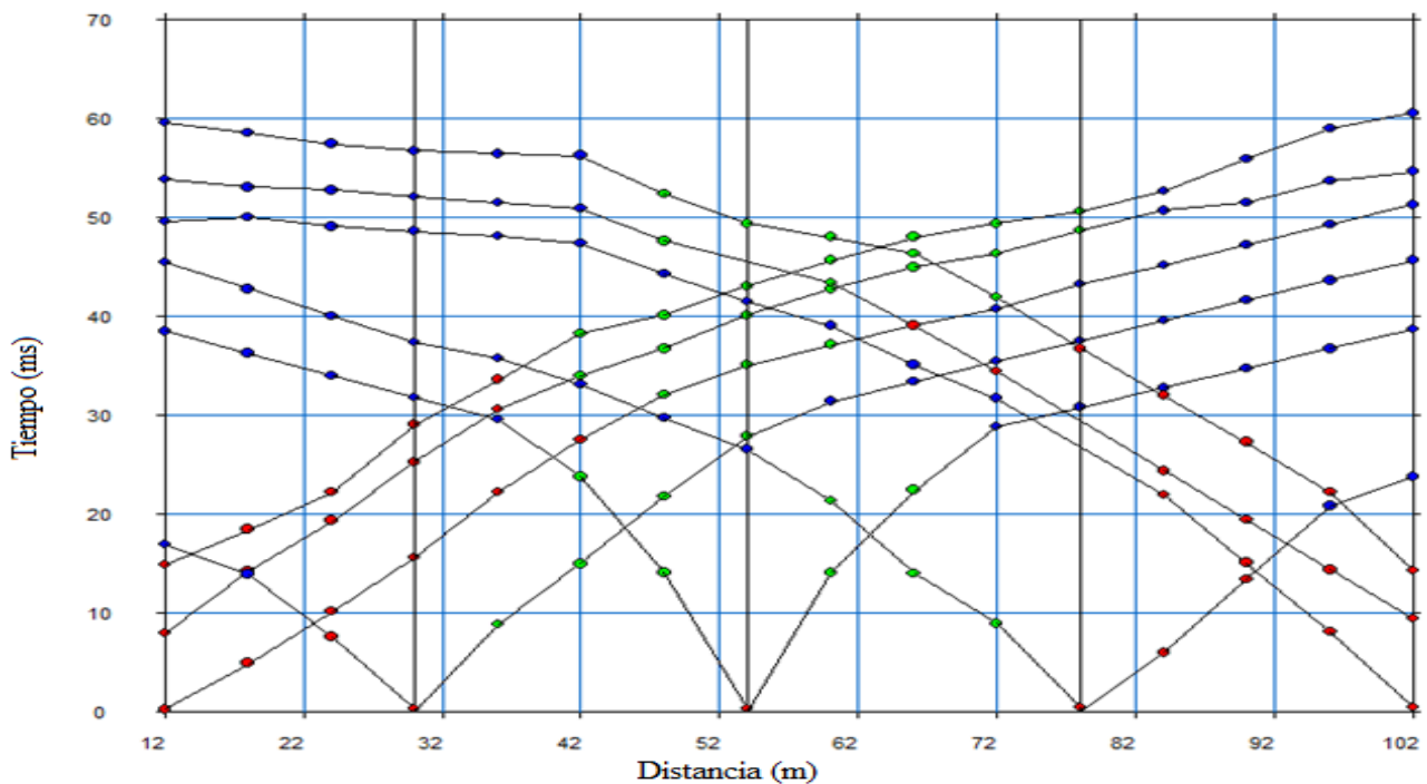
FIGURA 7: Datos crudos con los picados de los primeros arribos de todas las fuentes con una asignación de dos capas identificadas con los colores rojo y verde. Fuente: Autores.
