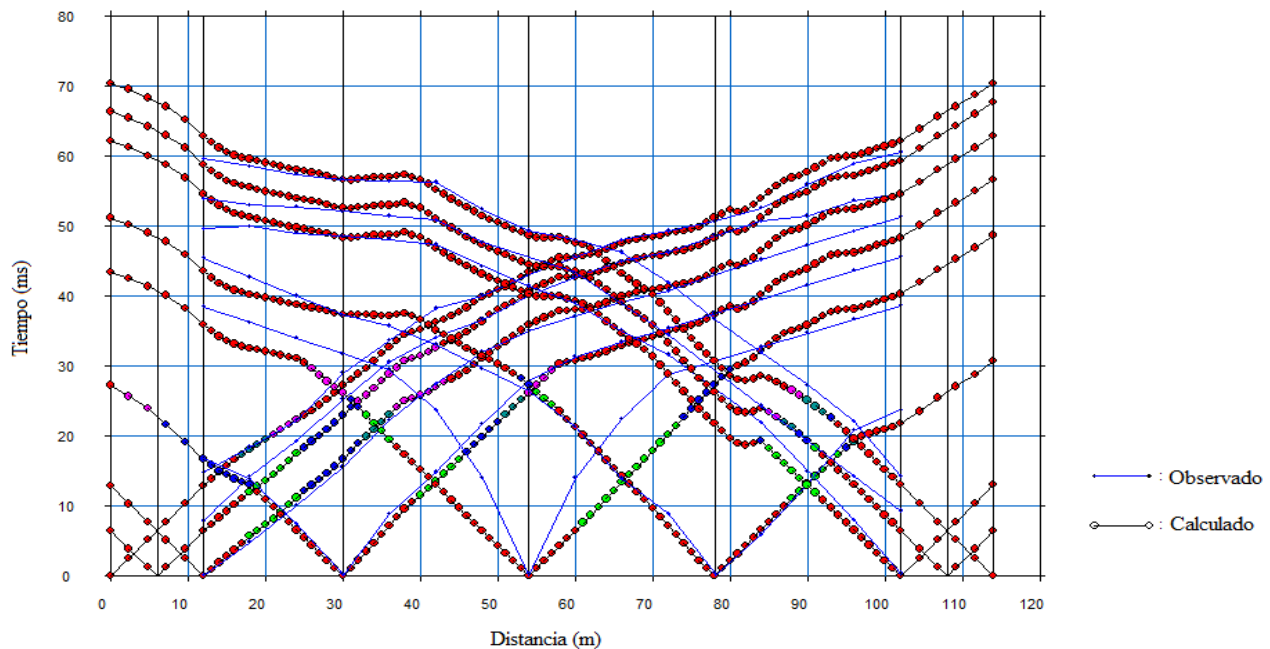
FIGURA 10: Curva de tiempo observado versus tiempo calculado para determinar el error del procedimiento. Fuente: Autores.
