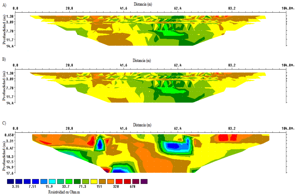
FIGURA 19: Pseudosecciones de resistividades aparentes. A) Pseudosección de resistividad aparente medida. B) Pseudosección de resistividad aparente calculada. C) Sección de resistividad del modelo del modelo de inversión. Fuente: Autores.
