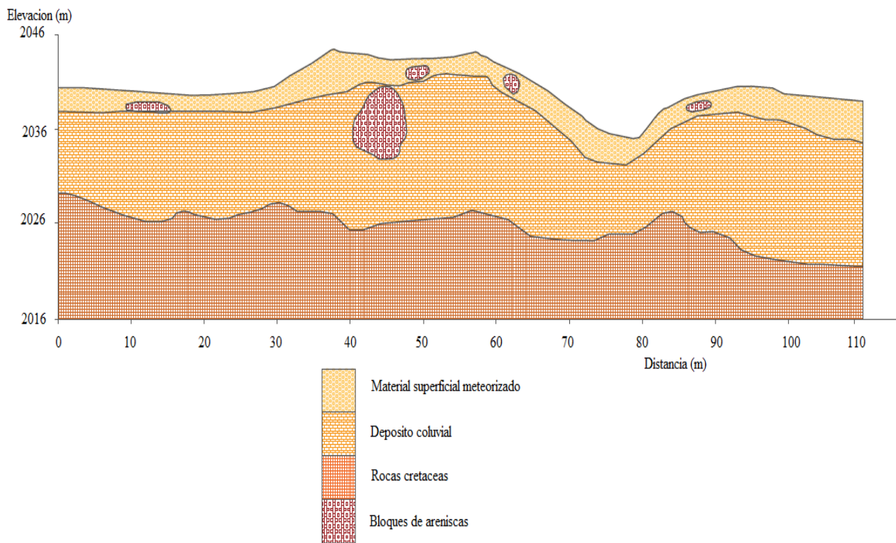
FIGURA 22: Perfil geológico obtenido con la relación de los tres ensayos analizados. Fuente: Autores.
