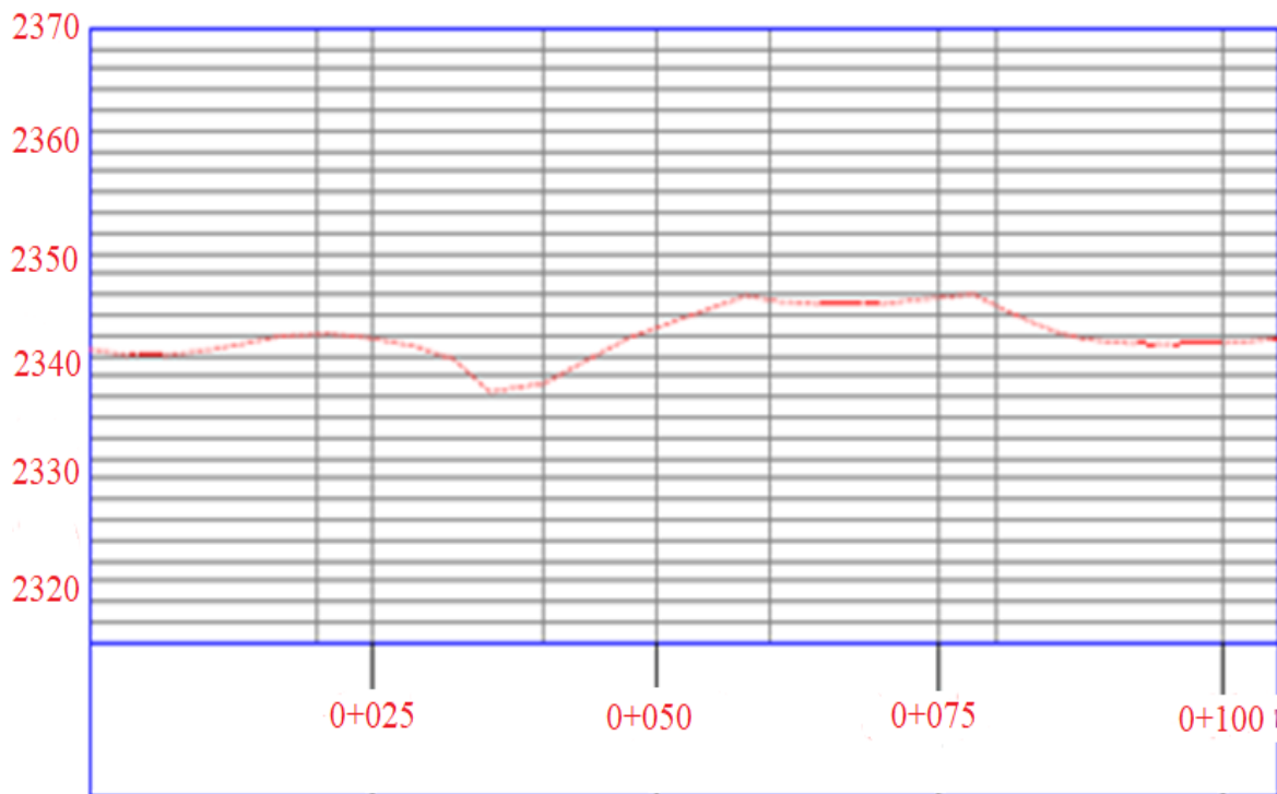
FIGURA 5: Perfil longitudinal de la línea de la Universidad de Pamplona. Fuente: Autores
