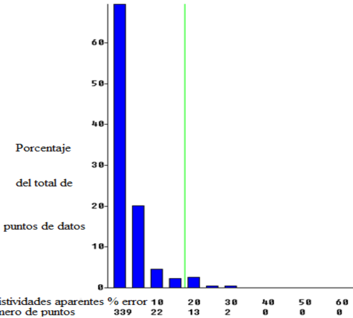
FIGURA 18: Porcentaje total de puntos dentro del 20 % de error de resistividades aparentes. Fuente: Autores.
