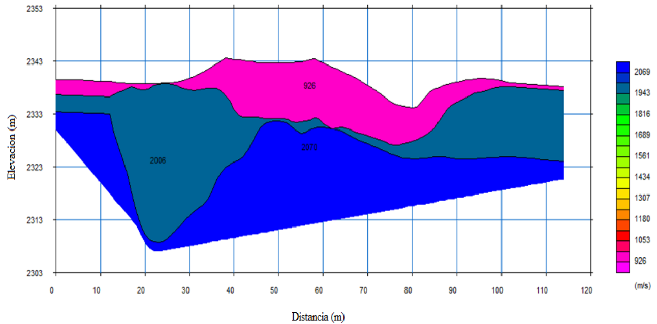
FIGURA 8: Modelo preliminar de inversión, con velocidades promedio en cada capa establecida. Fuente: Autores.
