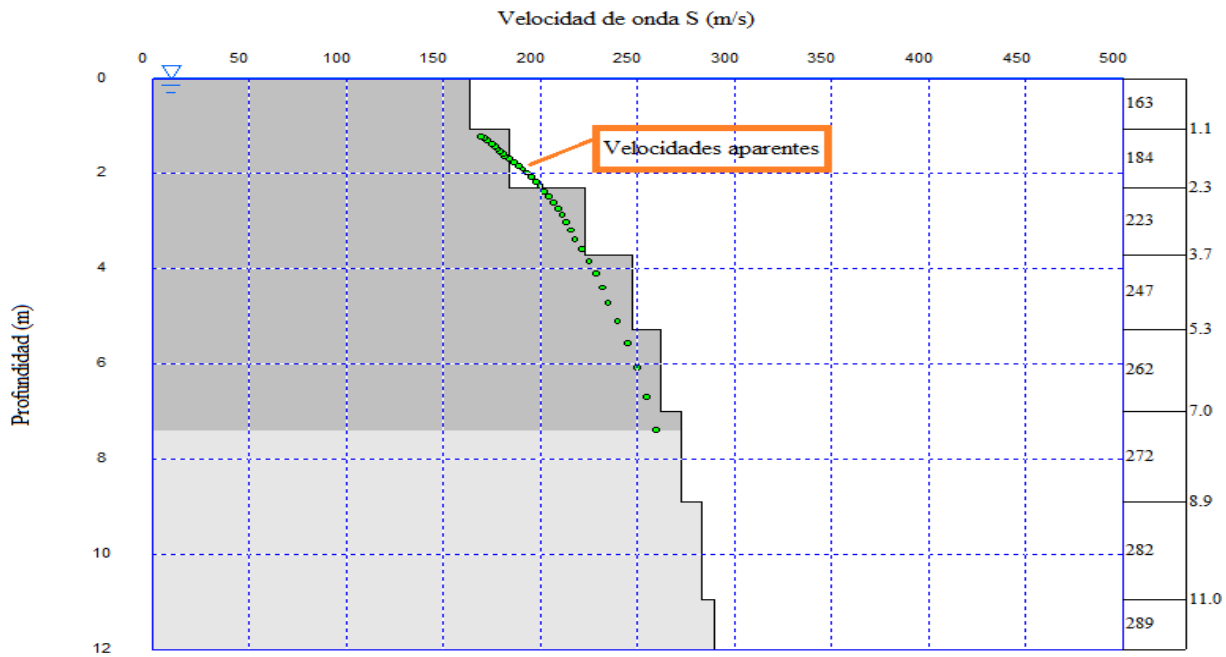
FIGURA 15: Modelo invertido de velocidades de onda S, con las velocidades aparentes punteadas en color verde. Fuente: Autores.
