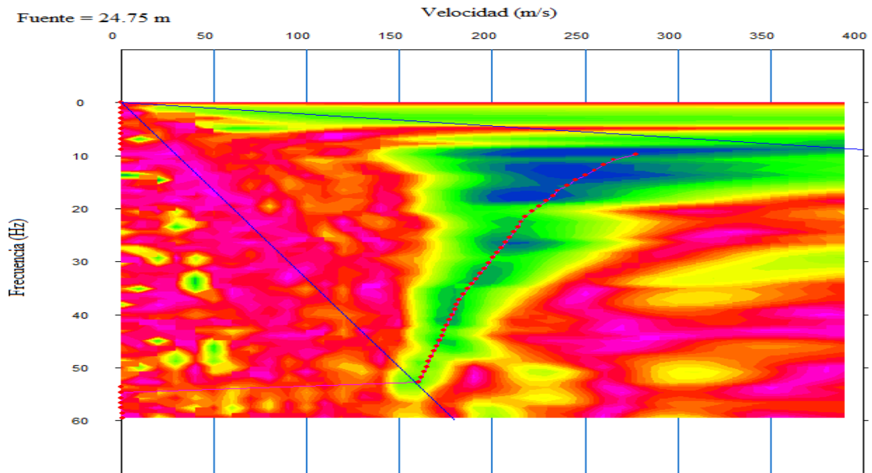
FIGURA 13: Curva de dispersión con sus respectivos picados (puntos rojos), pendiente de longitud de onda máxima (línea azul parte superior) y pendiente de longitud de onda mínima (línea azul parte inferior), para una fuente ubicada en la posición de 24.75 m del geófono 1. Fuente: Autores.
