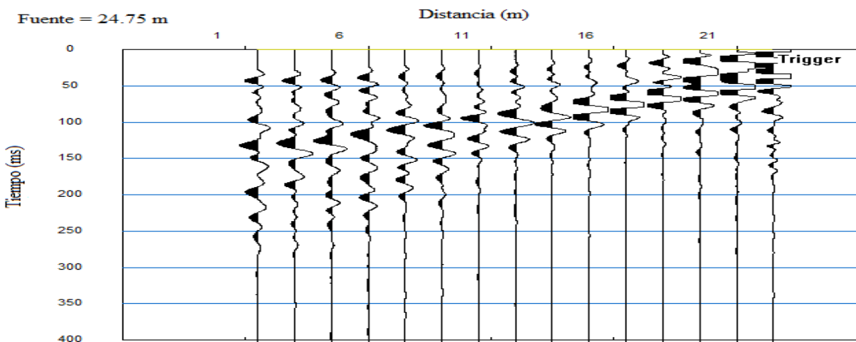
FIGURA 12: Dato crudo adquirido en campo, para una fuente ubicada en la posición de 24.75 del geófono 1. Fuente: Autores.
