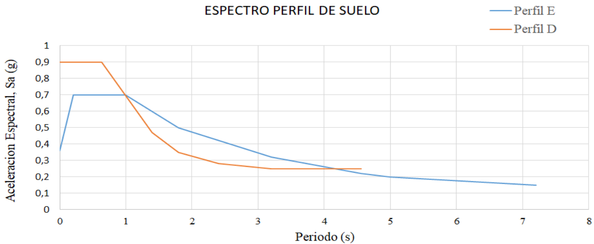
FIGURA 21: Espectro de los dos tipos de suelos obtenidos. Fuente: Autores.
