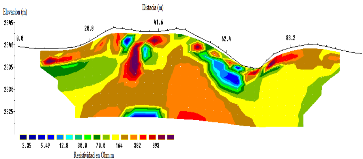
FIGURA 20: Modelo de resistividades reales con topografía. Fuente: Autores.
