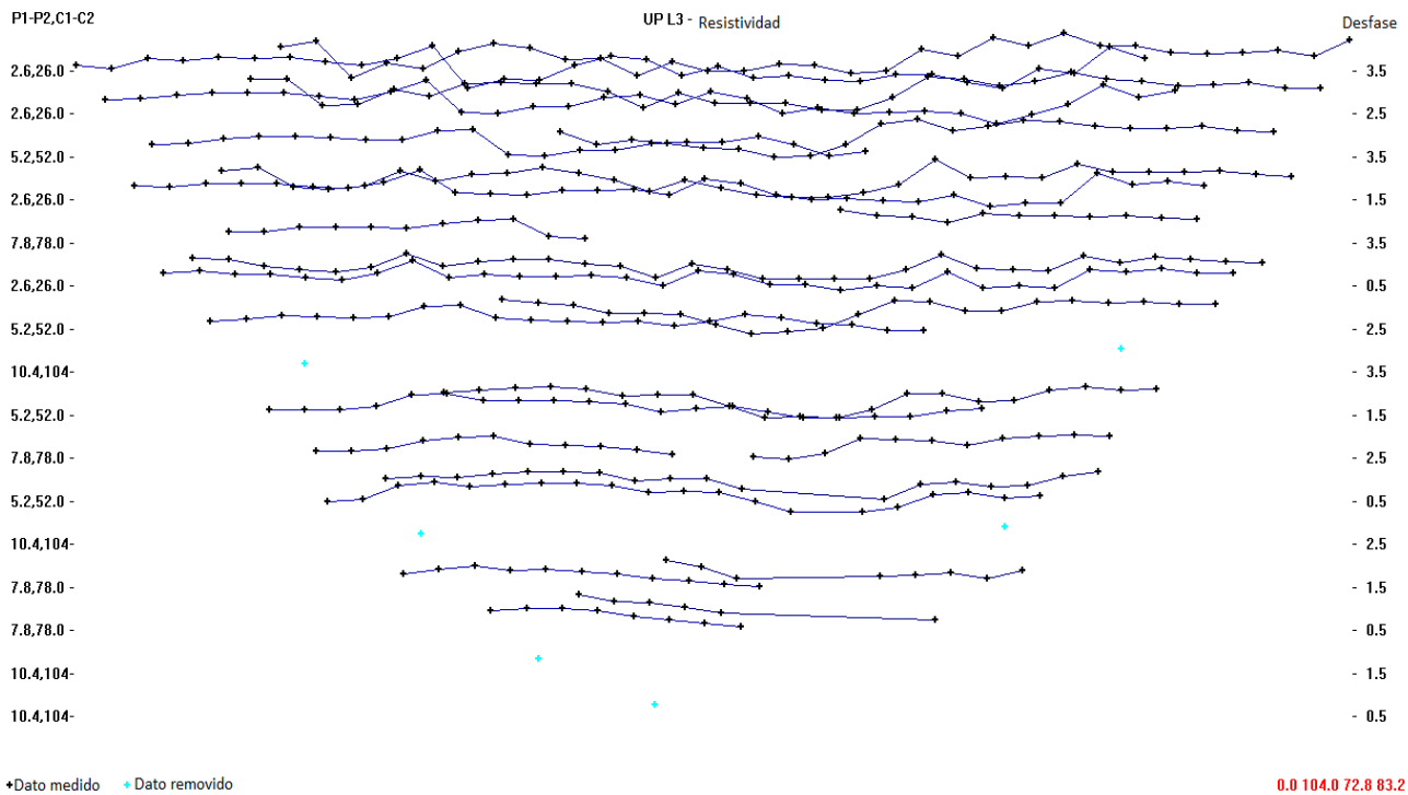
FIGURA 17: Distribución de puntos de datos de resistividad para eliminar puntos de datos malos en forma de perfiles. Fuente: Autores.
