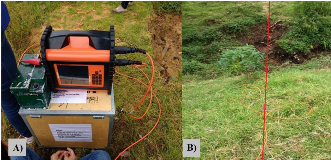
FIGURA 16: Adquisición de datos de métodos de geoelectrica. A) Equipo de adquisición de datos Terrameter LS (ABEM, 2012). B) Tendido de la línea con separación de electrodos de 2.6m. Fuente: Autores.
