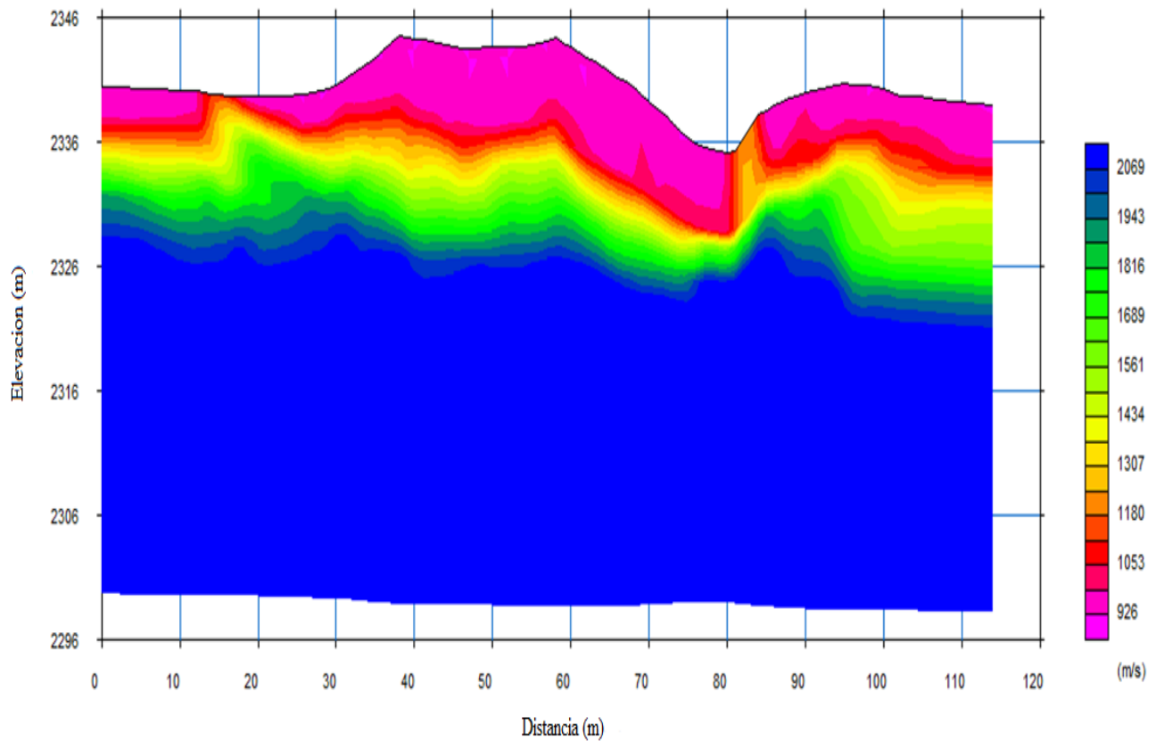
FIGURA 9: Modelo inversión por Tomografía Sísmica. Fuente: Autores
