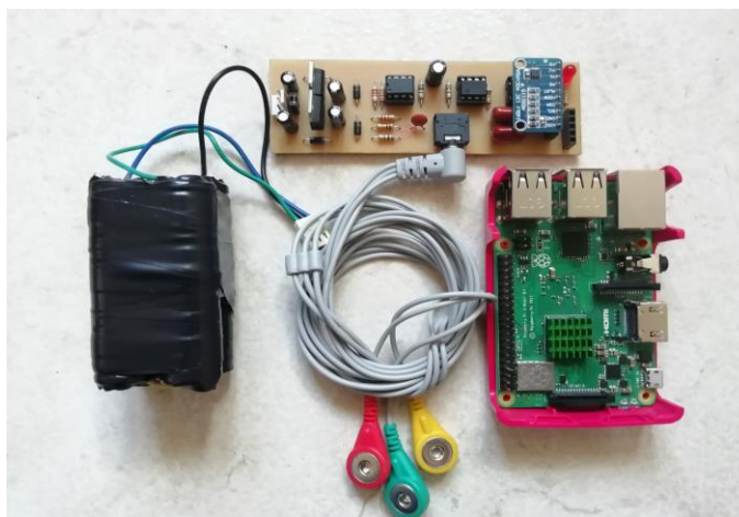
Figura 9. Implementación de circuitos finales. Fuente: Elaboración propia
