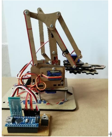
Figura 10. Sistema de control y brazo mecánico. Fuente: Elaboración propia
