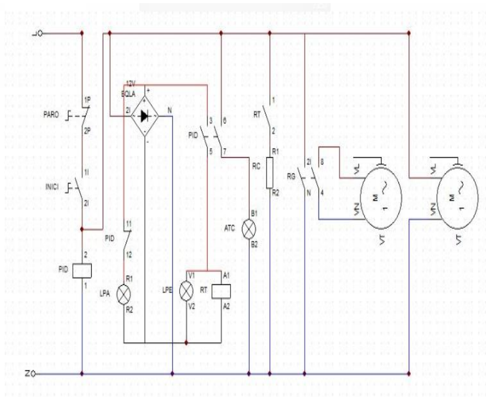
Plano 0.1 Diagrama electrico de la planta
