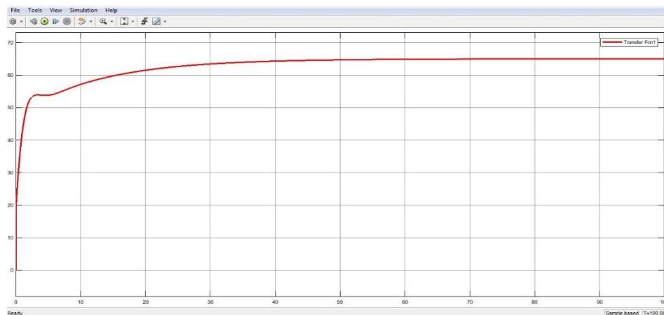
Figura 30: Comportamiento grafica control PID Autores
