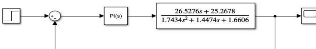
Figura 52: Diagrama retroalimentado control PI Autores
