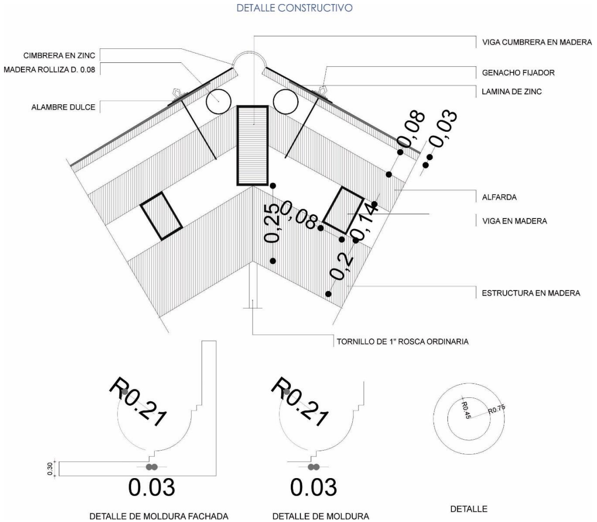
Ilustración 61. Detalle constructivo proyecto arquitectónico
