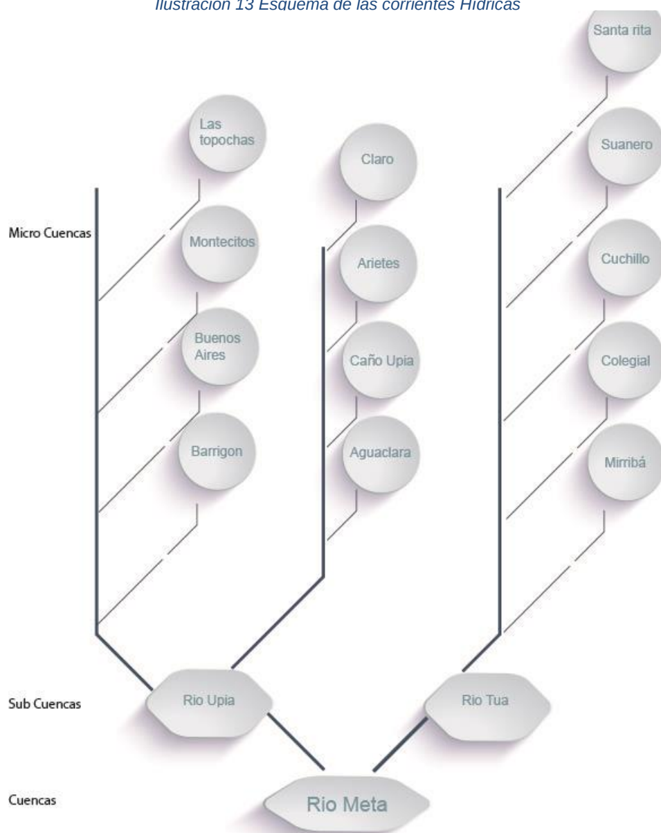
Ilustración 13 Esquema de las corrientes Hídricas
