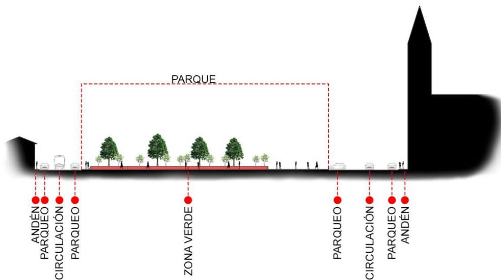
Ilustración 33 Corte Urbano parque Juana Escobar
