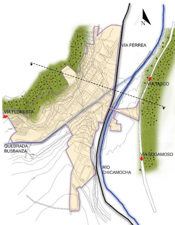
Ilustración 14 Topografía urbana Elaboración propia a partir del EOT
