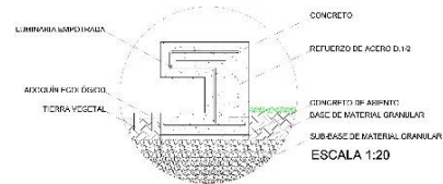
CORTE F-F"
