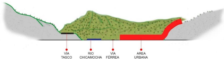
Ilustración 15 Corte urbano Elaboración propia
